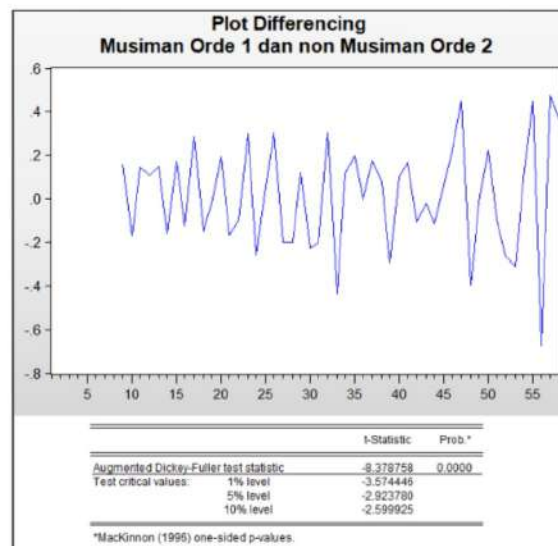
Gambar.3. Plot Data dan Output ADF test Hasil Transformasi dan Differencing
