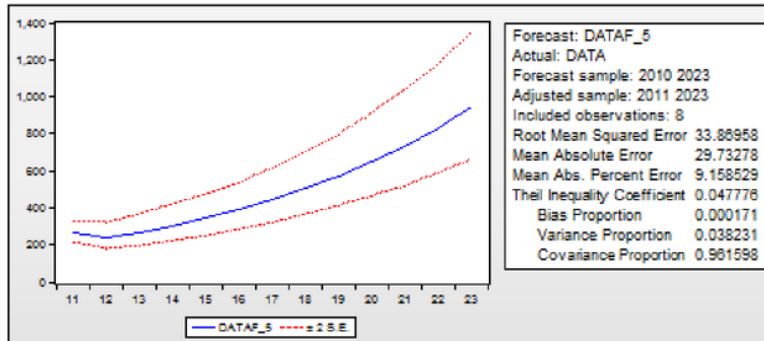
Gambar 6 : Grafik Peramalan Data Sampai 5 Periode Kedepan.
