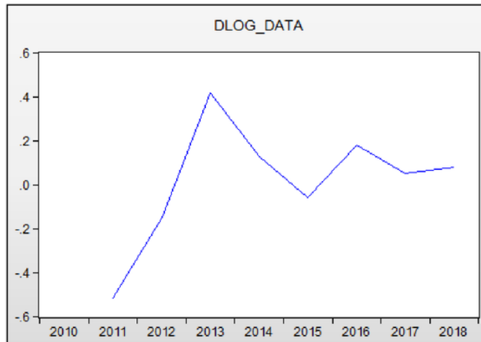
Gambar 3 : Grafik Hasil Differencing Setelah Data ditransformasi
